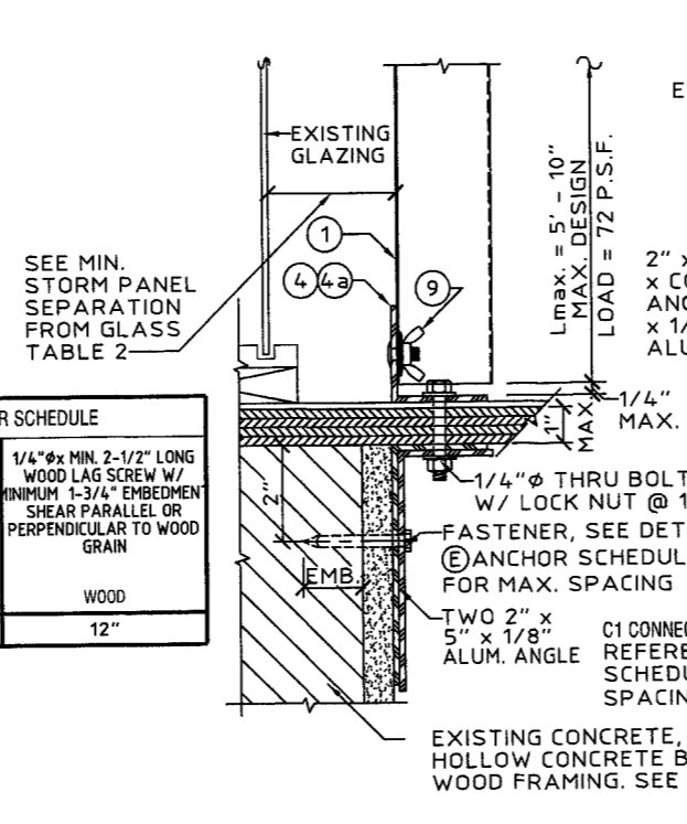
E) "PASS THRU" SECTION SCALE: 3" = 1' - 0"
